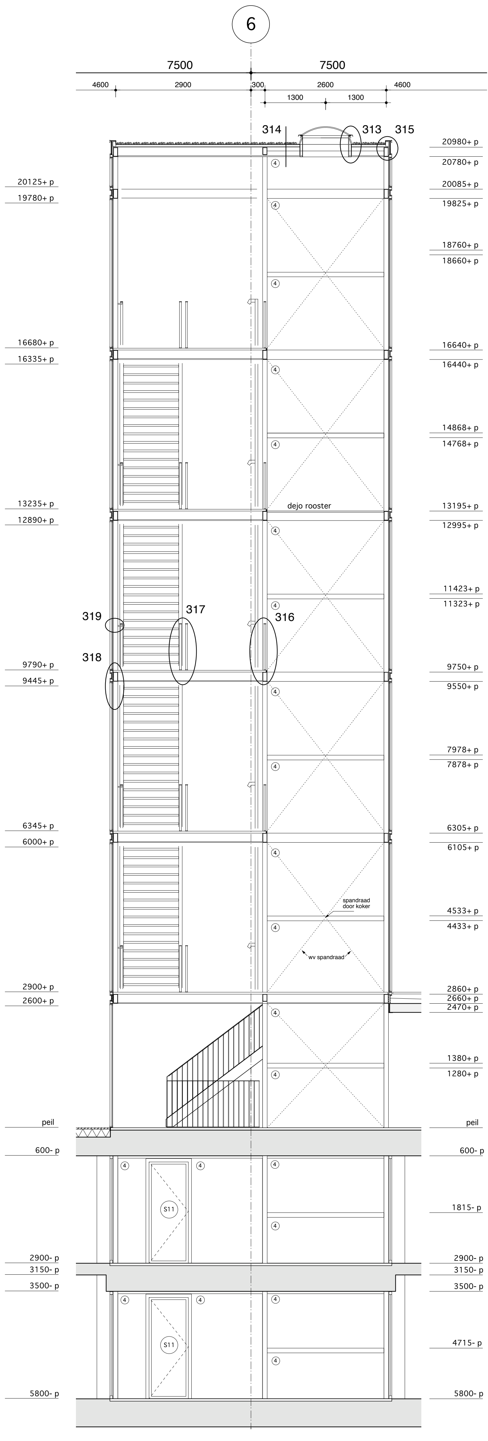
doorsnede Y
