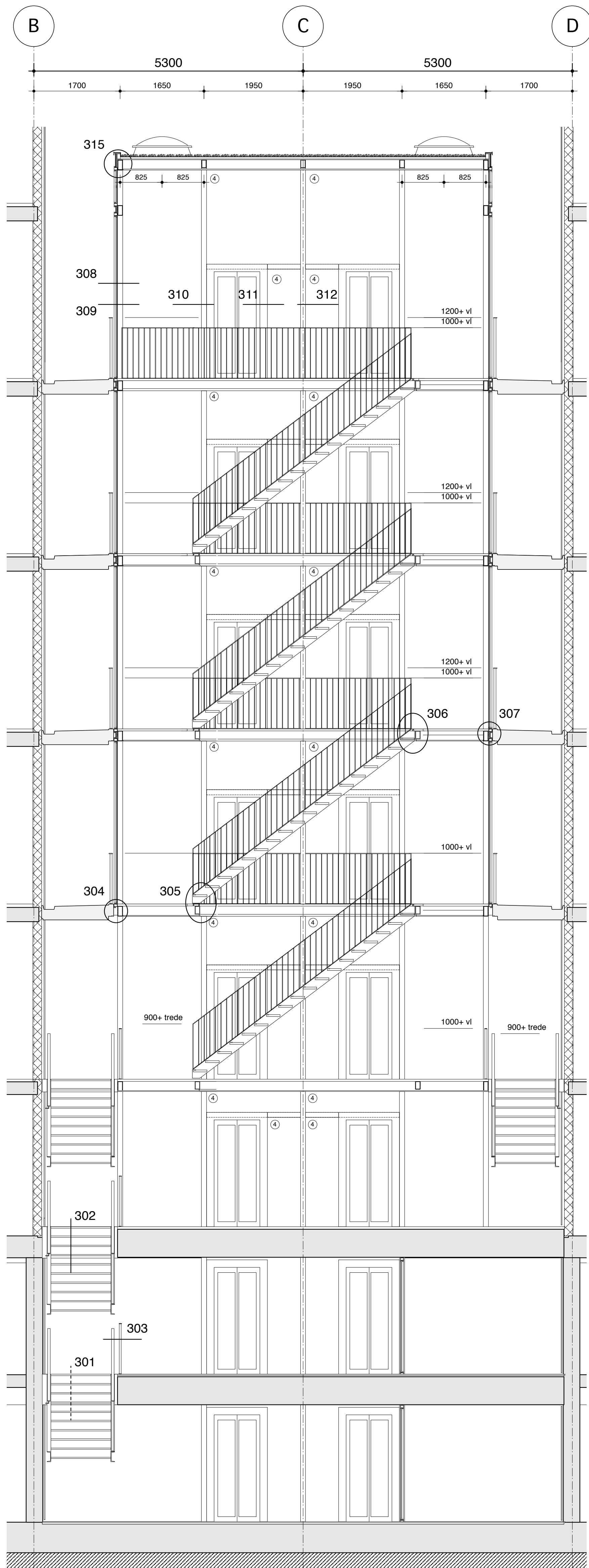
doorsnede X
