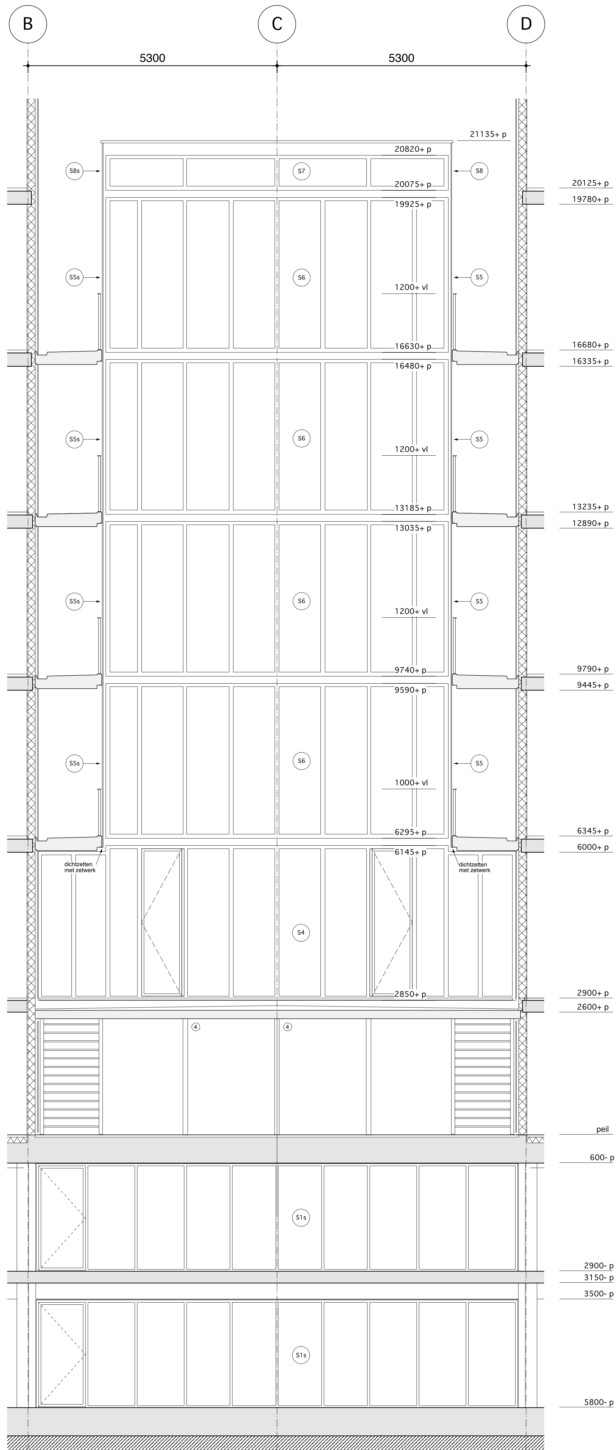
doorsnede V
